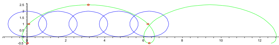
Figure 3: Rollkurve für einen Punkt außerhalb des Kreises
