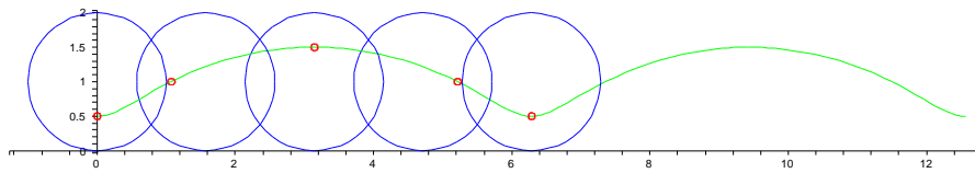
Figure 2: Rollkurve für einen Punkt innerhalb des Kreises
